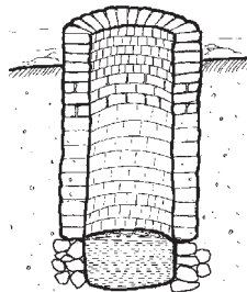
Guýynyň diwarlary boýdan-başa örülen
