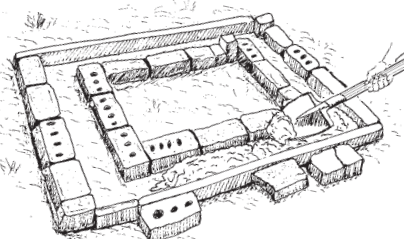
Betony ýerbe-ýer edip guýmak
