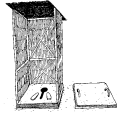
2 çukurlu kompost tuvaleti İnsan atıklarının gübre olarak kullanıldığı yerlerde tercih edilebilir.
