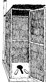
Havalandırılmalı çukur tuvalet Yeraltı suyunun derinde olduğu ve taşkın riskinin bulunmadığı yerlerde tercih edilebilir.
