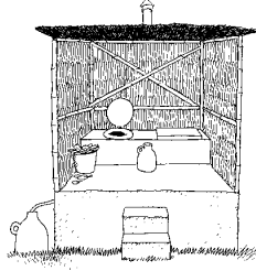
İdrarı ayıran kuru tuvalet İnsan atıklarının gübre olarak kullanıldığı, yeraltı suyunun yüksekte olduğu ya da taşkın riskinin bulunduğu yerlerde tercih edilebilir.
