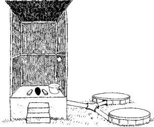
Sulu tuvalet Yeraltı suyunun derinde olduğu ve insanların dışkıladıktan sonra su kullandığı yerlerde tercih edilir.
